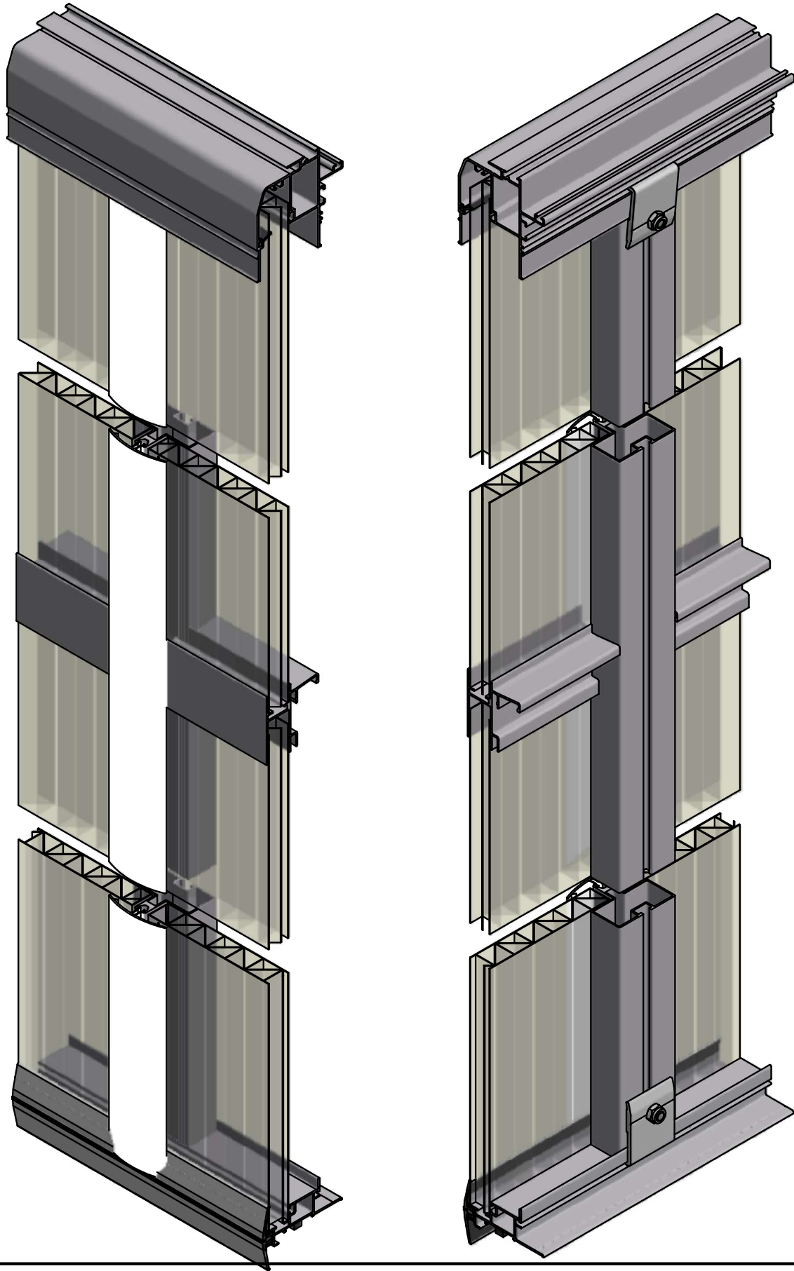
Title: Slimline greenhouse gable system (16mm SDP with panel divider) Slimline kasgevelsysteem (16mm SDP met steunregel)
